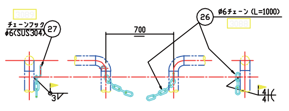
チェーンフック詳細
