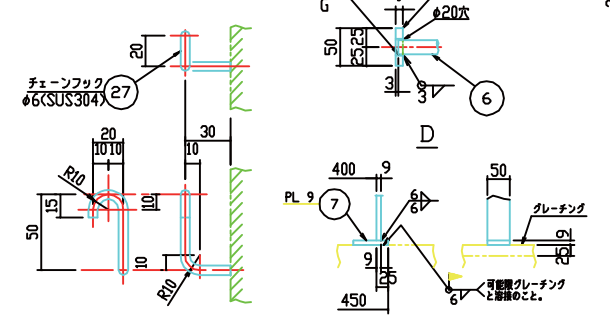
チェーンフック詳細
