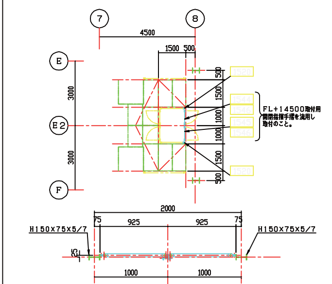
FL+4500 手摺改造配置図
