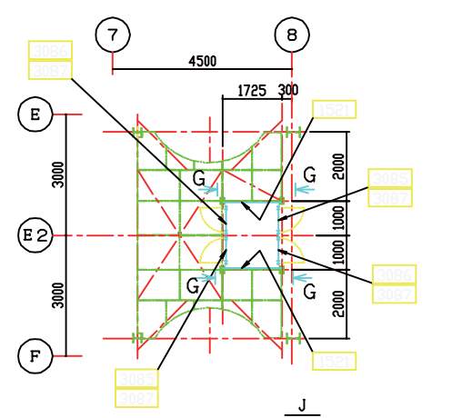
FL+14500 手摺改造配置図
