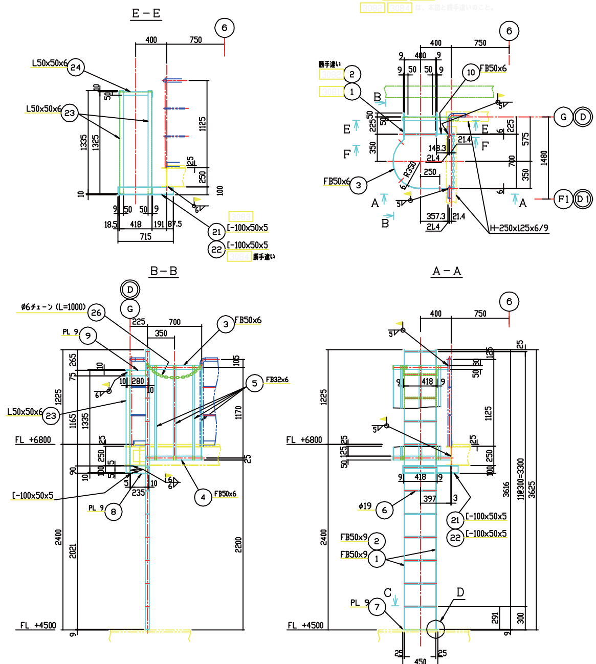
チェーン取付部詳細
