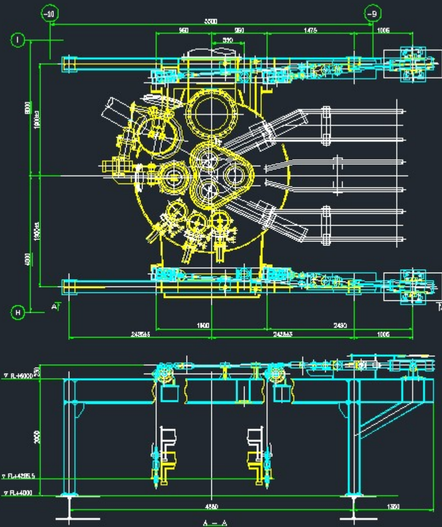
炉蓋吊上装置
