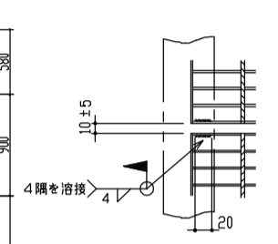
グレーチング取付要領
